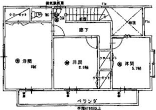
2F間取図
