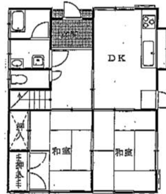
1F 平面図
