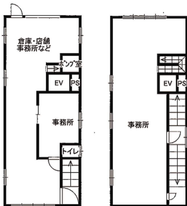
1F平面図
