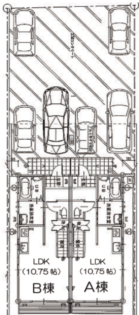
1F 平面図
