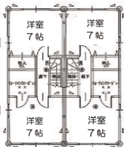
2F 平面図
