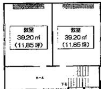
3F 平面図
